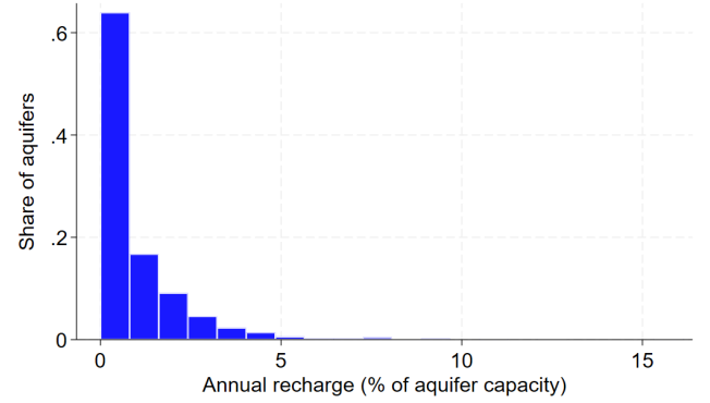
(d) Distribution of Annual Recharge
